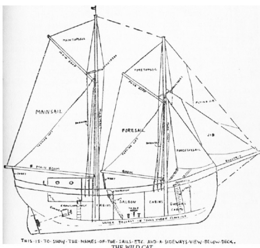
Divoká kočka (kresba AR)
